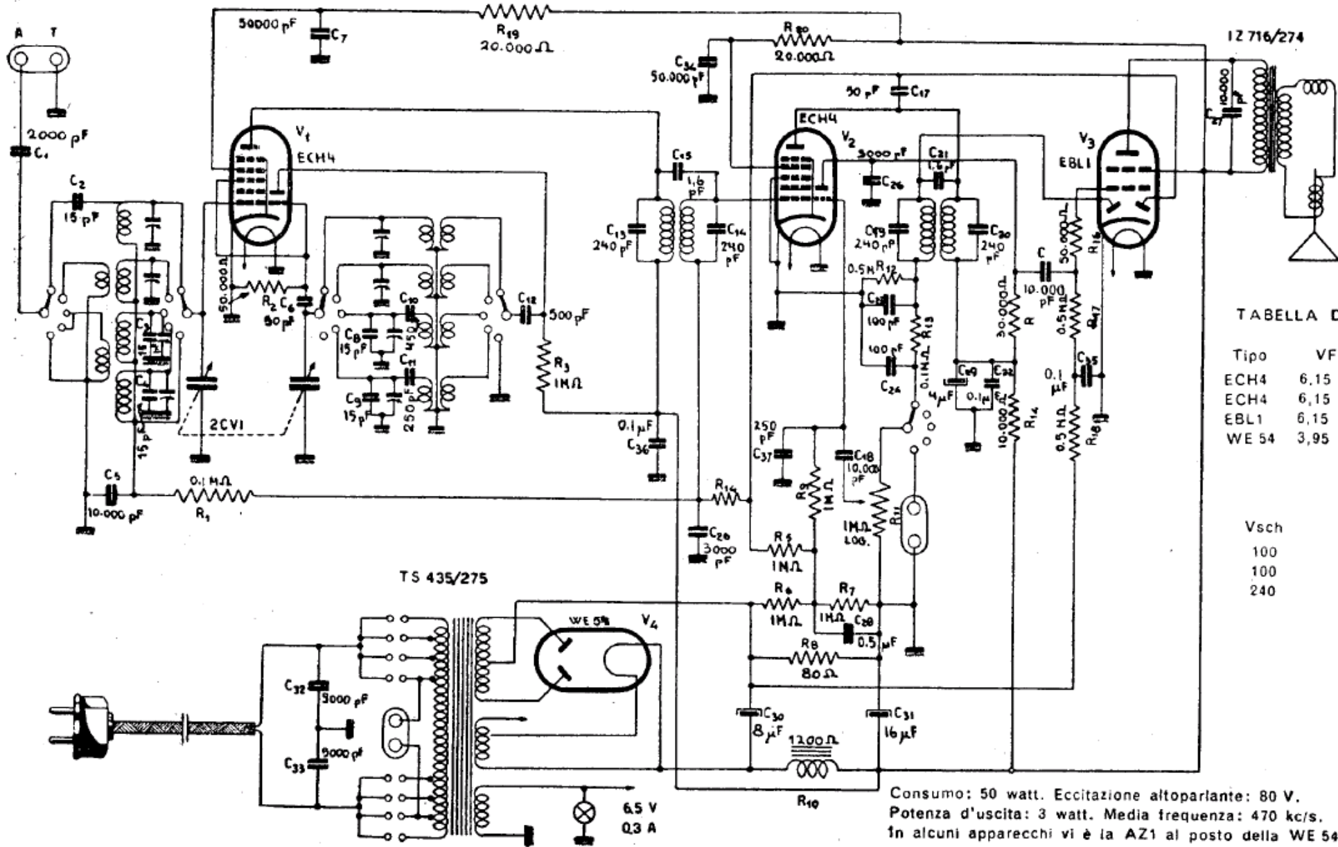
PHONOLA RADIO - Mod. 417 - Supereterodina con due ECH4, prima convertitrice, seconda amplificatrice MF e BF. Onde lunghe, medie, corte e cortissime. Media frequenza: 470 kc/s. Produzione 1945-46.
